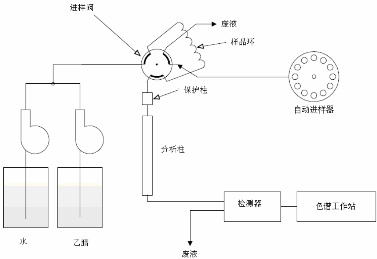
图 C.1 高效液相色谱系统的基本组成示意图
